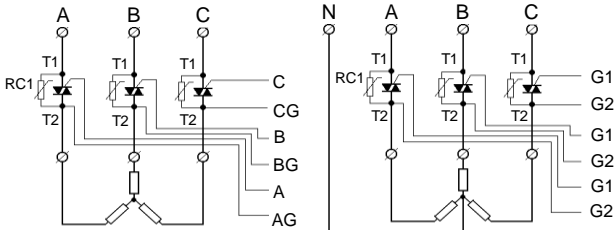
图 7: C5、K6 型应用 三相三线制移相触发
