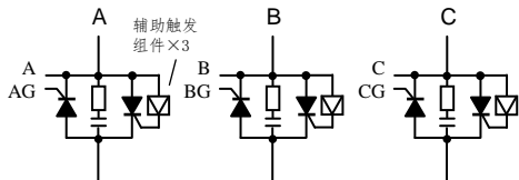
图 13: C7 型应用。单硅反并联，Y/Δ 接法。自动适应相序。 如果采用单硅和二极管反并联，则不按图中三个辅助组件
