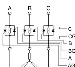
图 12: C5 型应用 三相三线制移相触发
