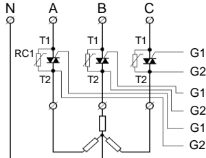
图 8: C4、K6 型应用 三相四线制移相触发
