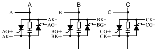
图 14: C8 全控型应用。单硅反并联，Y/Δ 接法。自动适应相序。
