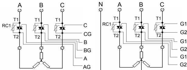
图 7: C5、K6 型应用三相三线制移相触发
