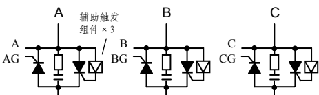
图 13: C7 型应用。单硅反并联，Y/Δ 接法。自动适应相序。如果采用单硅和二极管反并联，则不按图中三个辅助组件
