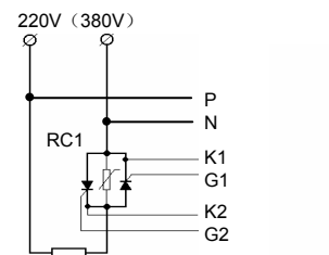
图 11: C2 型应用二相触发电型单路移相触发
