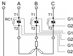
图 8: C4、K6 型应用三相四线制移相触发
