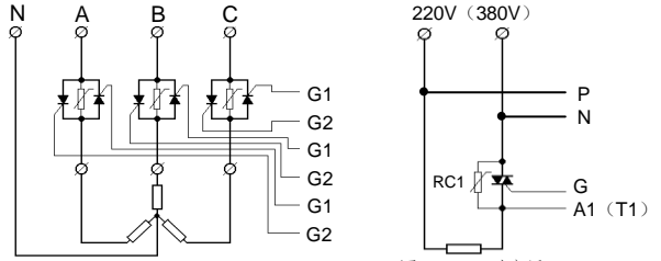
图 9: C4、K6 型应用 三相四线制移相触发
