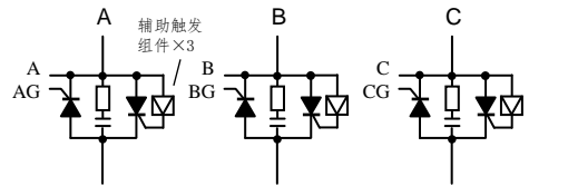
图 13: C7 型应用。单硅反并联, Y/Δ 形接法。自动适应相序。如果采用单硅和二极管反并联, 则不按图中三个辅助组件
