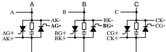
图 14: C8 全控型应用。单硅反并联, Y/Δ 形接法。自动适应相序。
