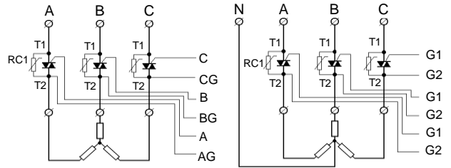
图 7: C5、K6 型应用 三相三线制移相触发
