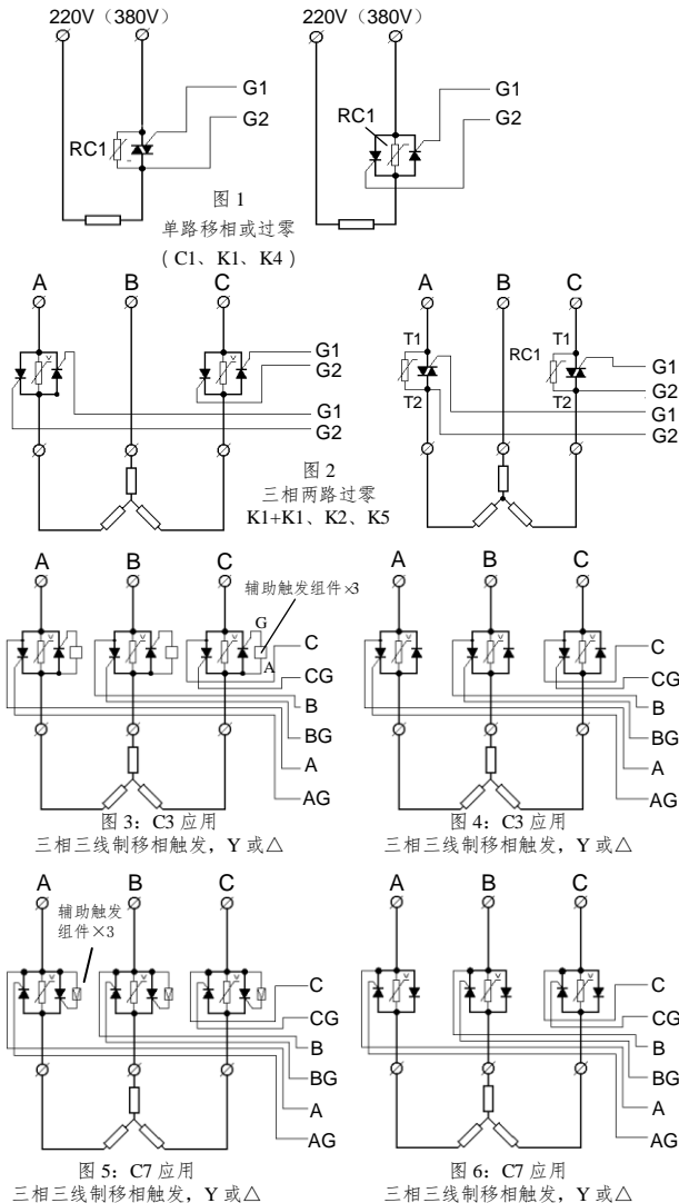
图 13: C7 型应用。单硅反并联, Y/Δ 形接法。自动适应相序。如果采用单硅和二极管反并联, 则不按图中三个辅助组件
