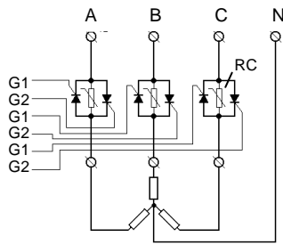
图 24 C4、K6 接线
