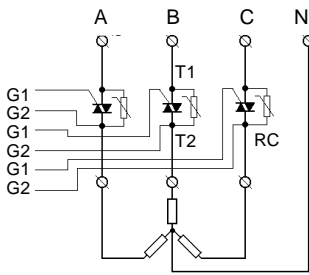
图 23 C4、K6 接线
