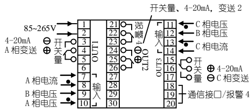
附：三相三线制接线图（修改接线方式必须重新上电后生效！）
