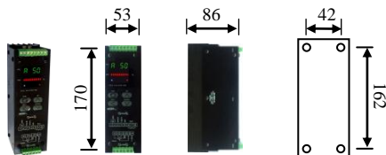
3.1 单相 5~20A 安装尺寸
