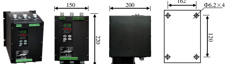
3.7 三相 100~140A 安装尺寸:
