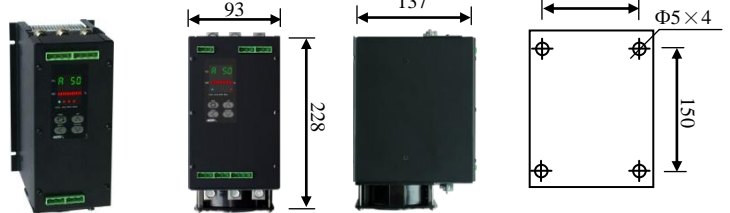
3.6 三相 60~90A 安装尺寸:
