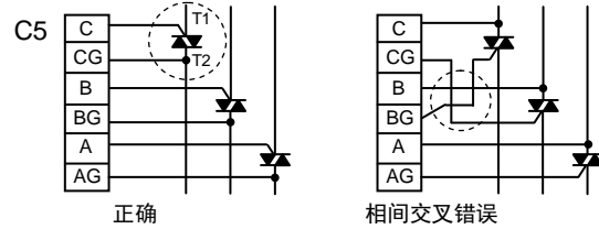
正确 相间交叉错误
