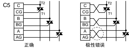
正确 极性错误
