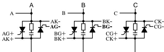
图 13: C8 全型应用。单硅反并联, Y/ \Delta 形接法。自动适应相序。
