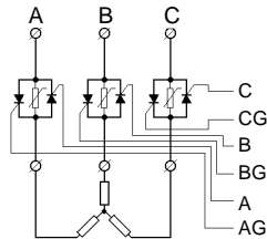
图 6: C5 应用 三相三线制移相触发, Y 或 \Delta
