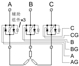
图 5: C7 应用。三相三线制移相触发, Y 或 \Delta 。如果采用单硅和二极管反并联, 则不接图中三个辅助组件
