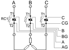
图 7: C5、K6 型应用 三相三线制移相触发
