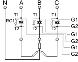
图 8: C4、K6 型应用 三相四线制移相触发
