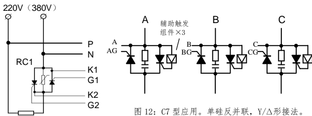
图 11: C2 型应用二 传统触发型单路移相触发
