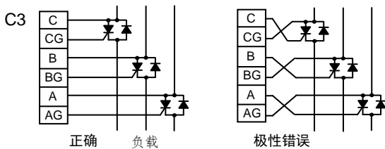
正确 负载 极性错误
