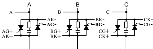
图 16: C8 全控型应用。单硅反并联, Y/□形接法。自动适应相序。
