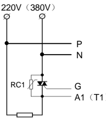
图 10: C2 型应用一 传统触发型单路移相触发
