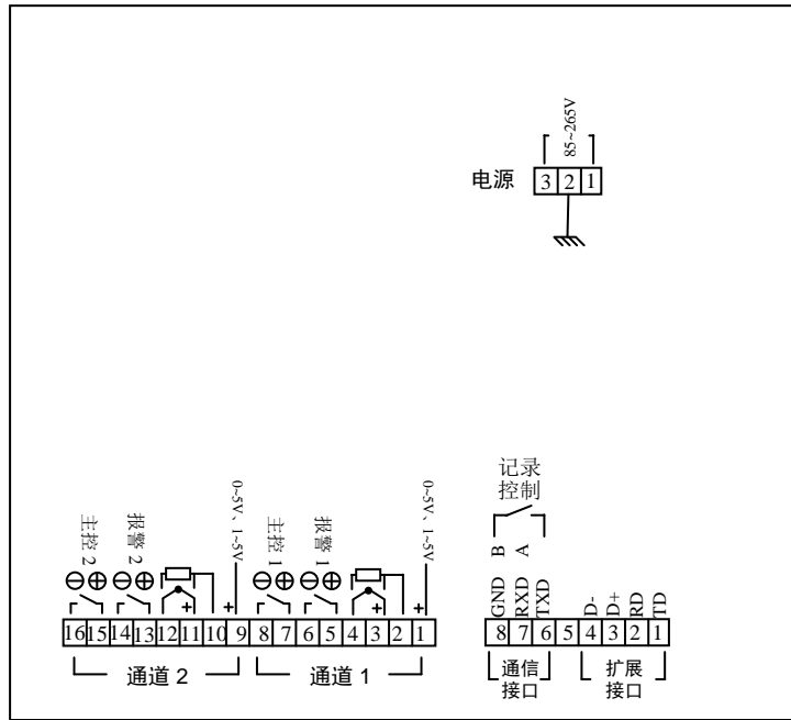
图 4.4 1-2 (L1 外形尺寸) 通道产品接线端子排布
