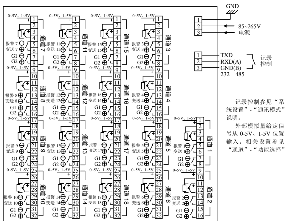
图 4.2 15-18(L3 外形尺寸)通道产品接线端子排布
