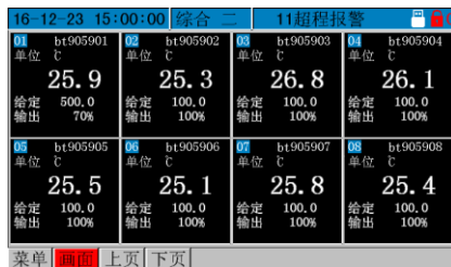
图 5.7 综合数显画面三
