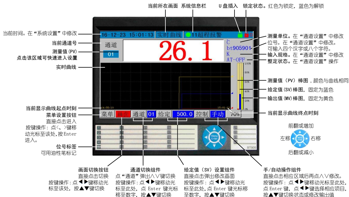
图 5.1 实时曲线画面
