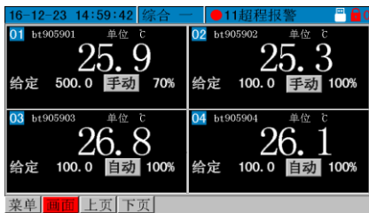
图 5.6 综合数显画面二
