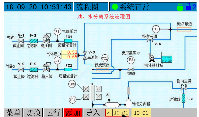
图 24 出现开关状态控件
