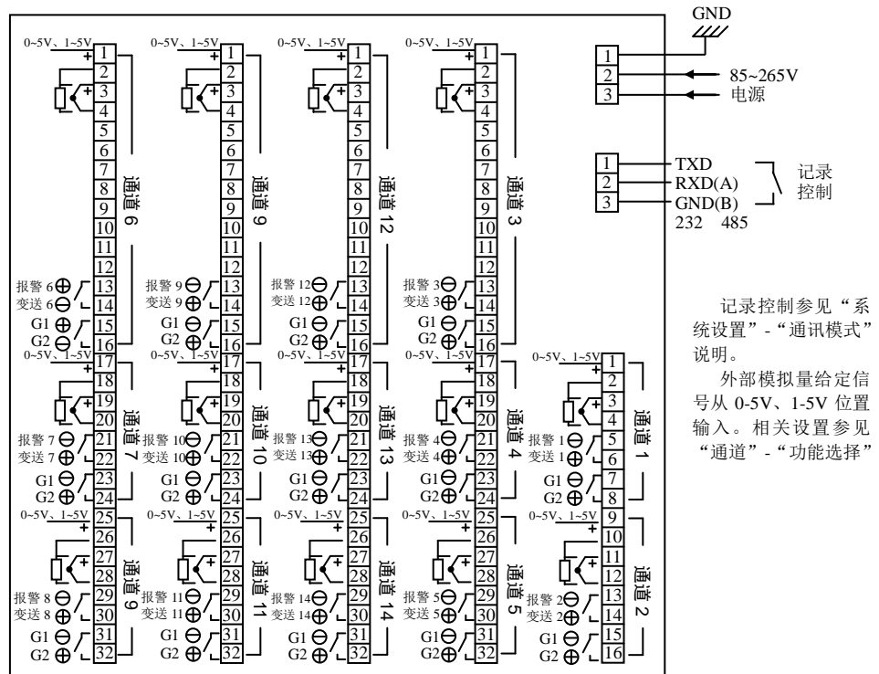
图 4.3 3-14 (L2 外形尺寸) 通道产品接线端子排布
