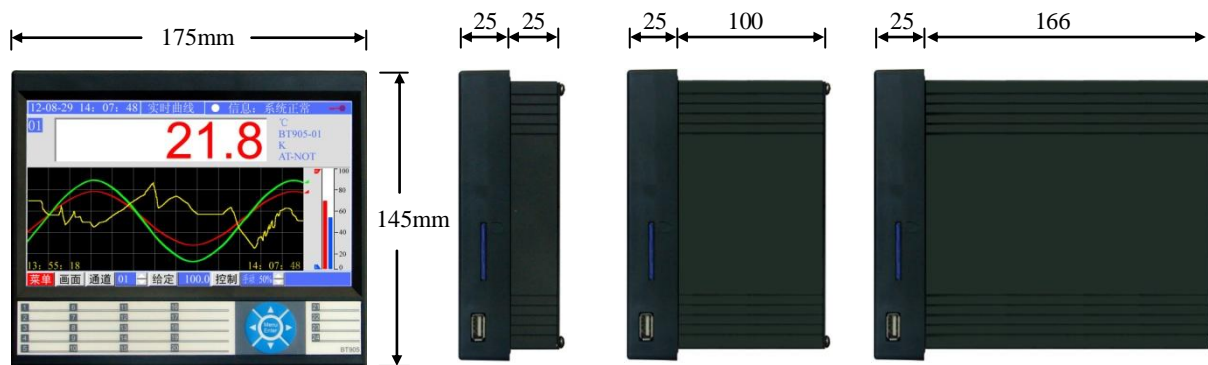
图 4.1 正面视图
