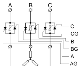
图 12: C3 型应用 三相三线制移相触发
