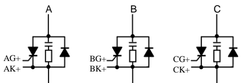
图 13: C6 半控型应用。单硅二极管反并联，Y/Δ形接法。自动适应相序。 如果采用单硅和二极管反并联，则不按图中三个辅助组件
