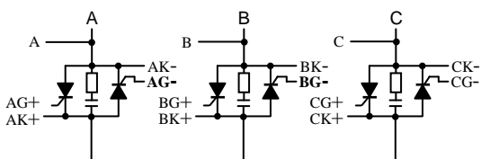
图 14: C8 全控型应用。单硅反并联，Y/Δ形接法。自动适应相序
