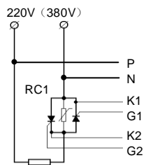
图 11: C2 型应用二 传统触发型单相移相触发
