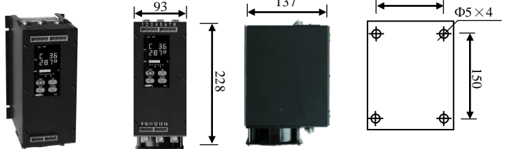
3.6 三相 60~90A 或单相 200~250A 安装尺寸:
