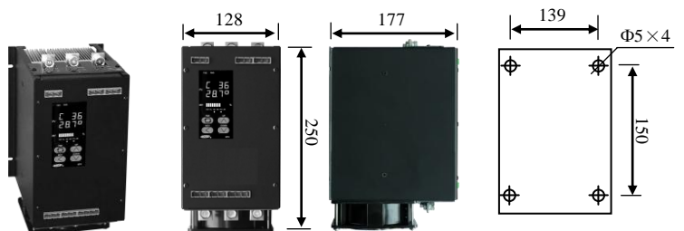
3.6 三相 60~90A 或单相 200~250A 安装尺寸:
