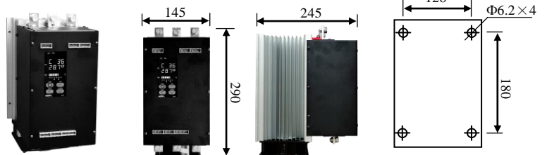
3.8 三相 150~190A 安装尺寸:
